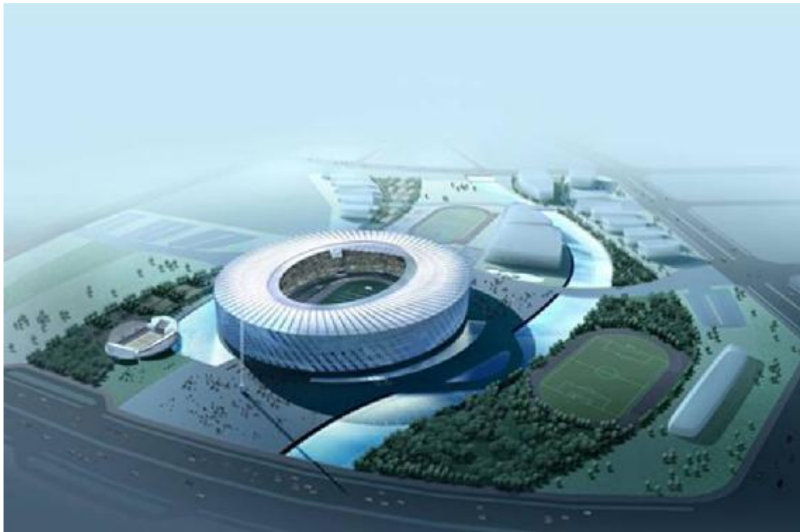
广东省惠州市中心体育场是举办2010年第十三届省运会的主会场。建筑设计以“盛世舞台”为理念,采用岭南客家围屋和客家斗笠的造型,体现人文、绿色、和谐的主题和惠州本土文化气息。总建筑面积62056平方米,可容纳4万多名观众。惠州市中心体育场棚架结构为空间管桁架结构,总用钢量8650吨。本工程铸钢节点与相邻节点相接口多达11个,在铸钢件几何尺寸精度要求上相当高。
